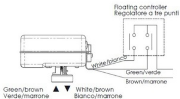
collegamento a 3 punti / 3-point connection
